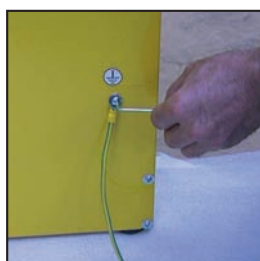
Vite di fissaggio a brugola 5 mm per attacco messa a terra.
